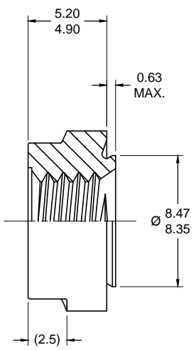
SECTION A-A SCALE 3:1
